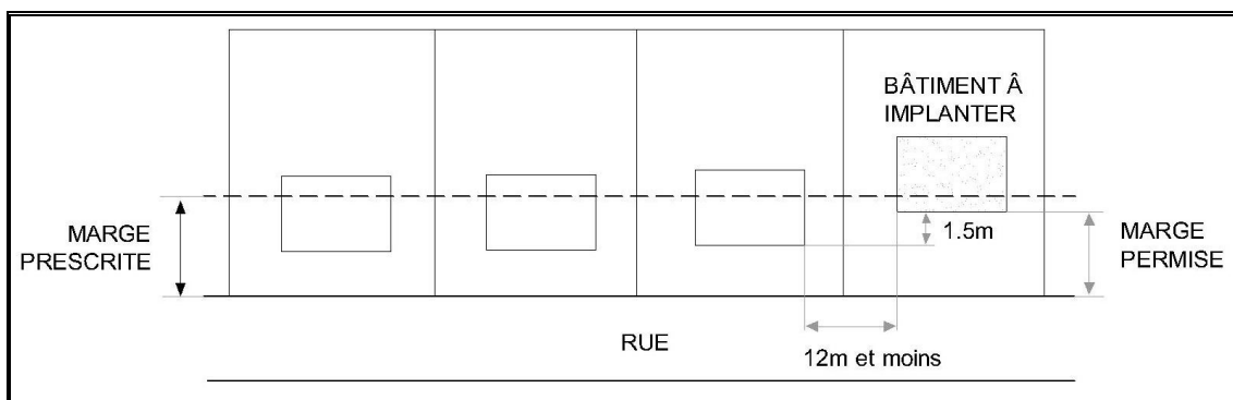
CROQUIS 27 : IMPLANTATION A LA SUITE DU DERNIER BATIMENT PRINCIPAL EXISTANT
